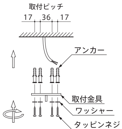
図2 A部取付詳細
