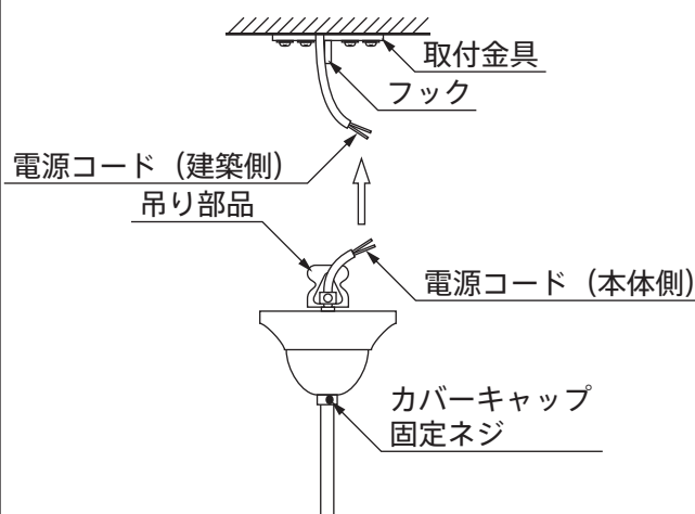
図3 A部取付詳細
