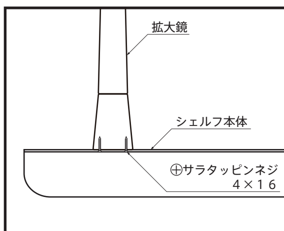
●取付断面図
