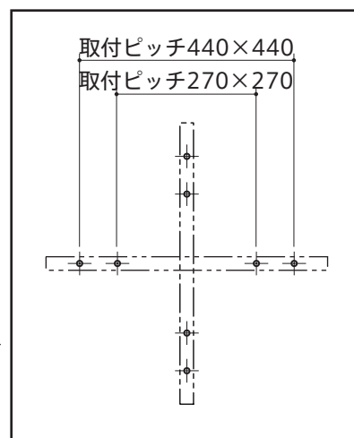
取付け金具固定位置
