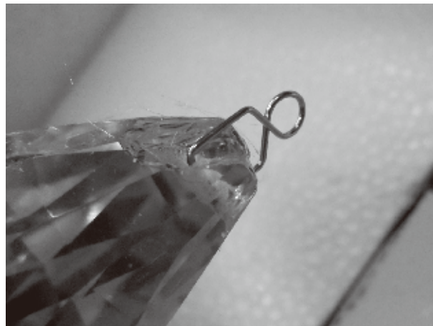
■オーナメント取付部分詳細
