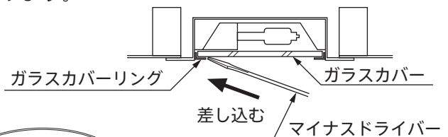
断面詳細図
