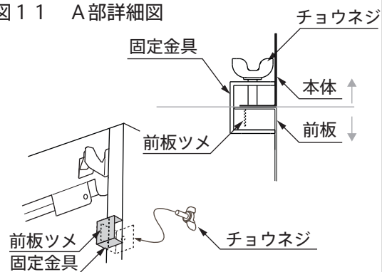
図11 A部詳細図
