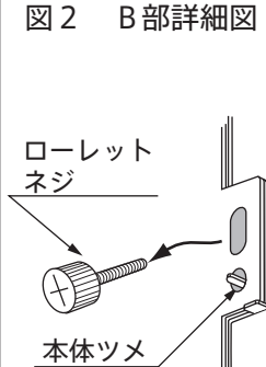
図2 B部詳細図
