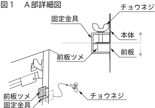
図1 A部詳細図
