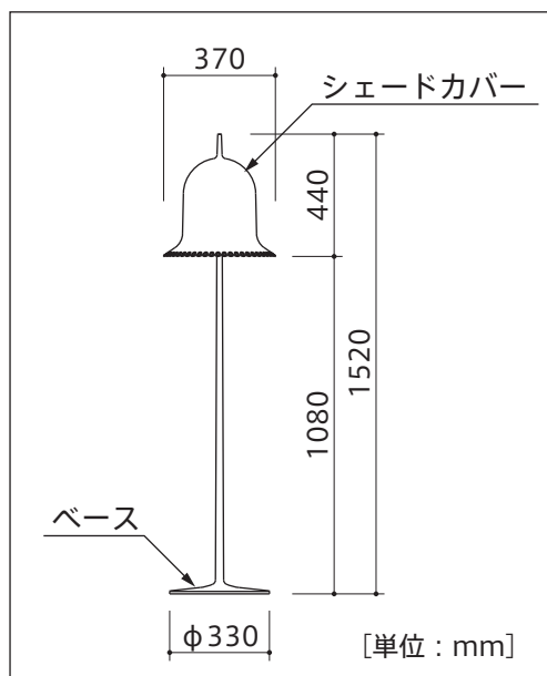
■製品寸法図
