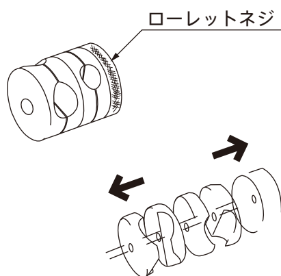
図5 クランプ
