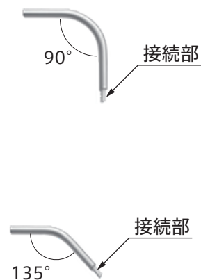
図 4 ジョイント金具
