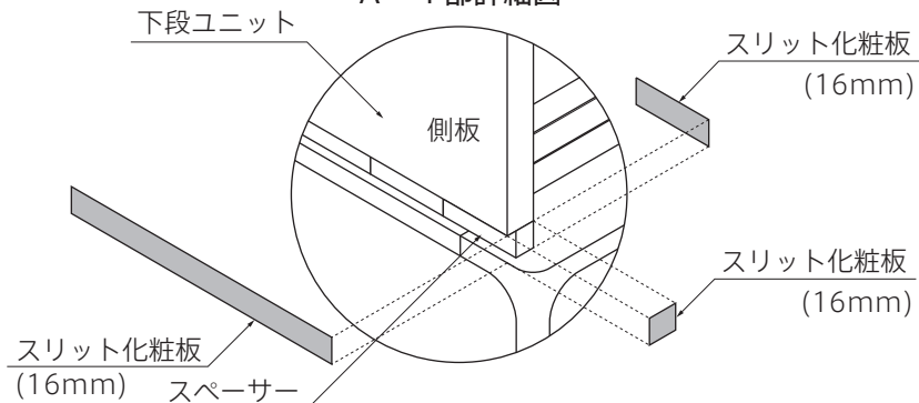
A-1 部詳細図
