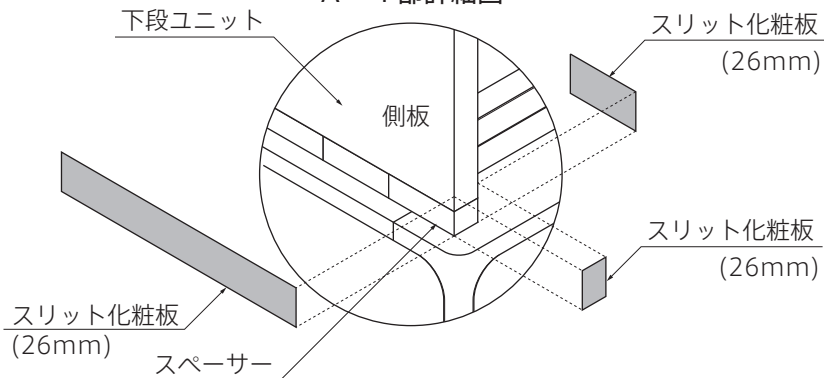
A-1 部詳細図
