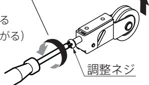
図1 上部ローラー
