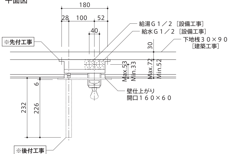
平面図
