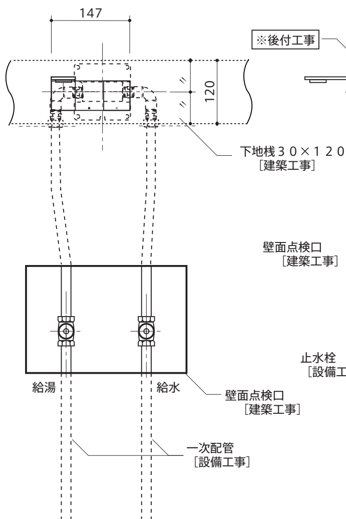
側面図
