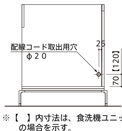
側面図（側板に穴を開ける場合）
