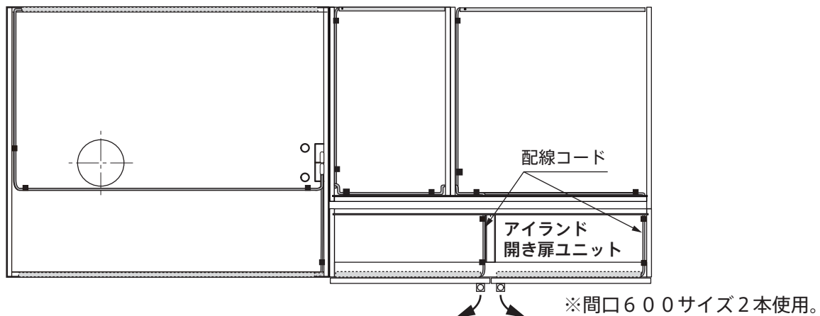
正面図
