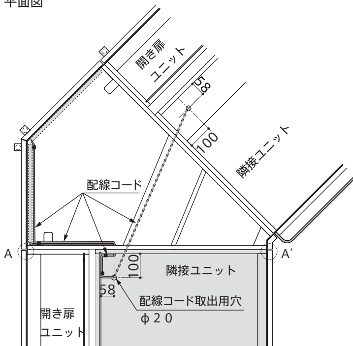
平面図
