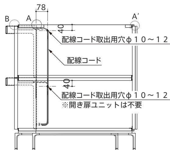
側面図
