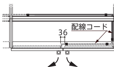
平面図
