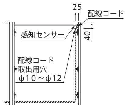
正面図
