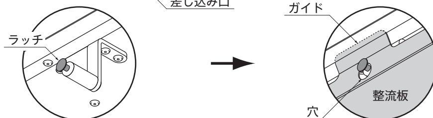
B部詳細図
