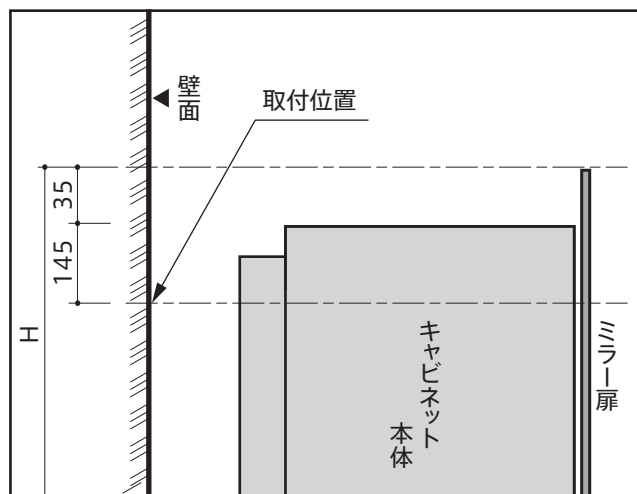
取付位置の側面図
