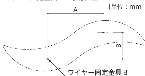
ワイヤー固定金具B 取付位置
