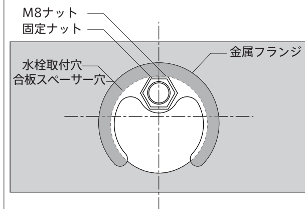
図5 天板裏面から見た取付位置
