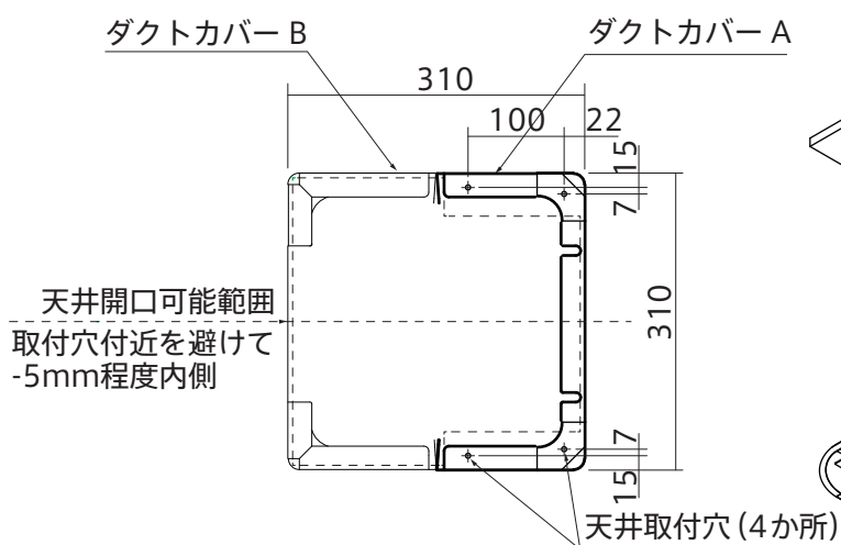
上面図 1/10
