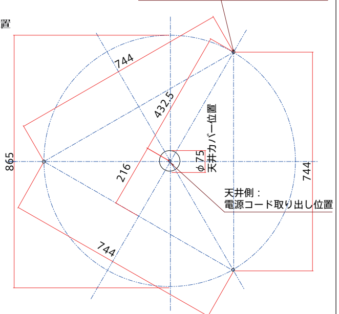
SFHL - CALIPSO - 100 天井吊り位置 <見上げ図>参考
