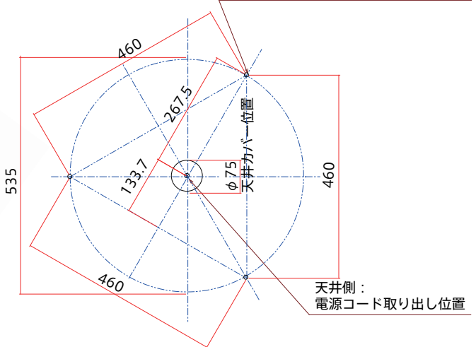
SFHL - CALIPSO - 65 天井吊り位置 <見上げ図>参考
