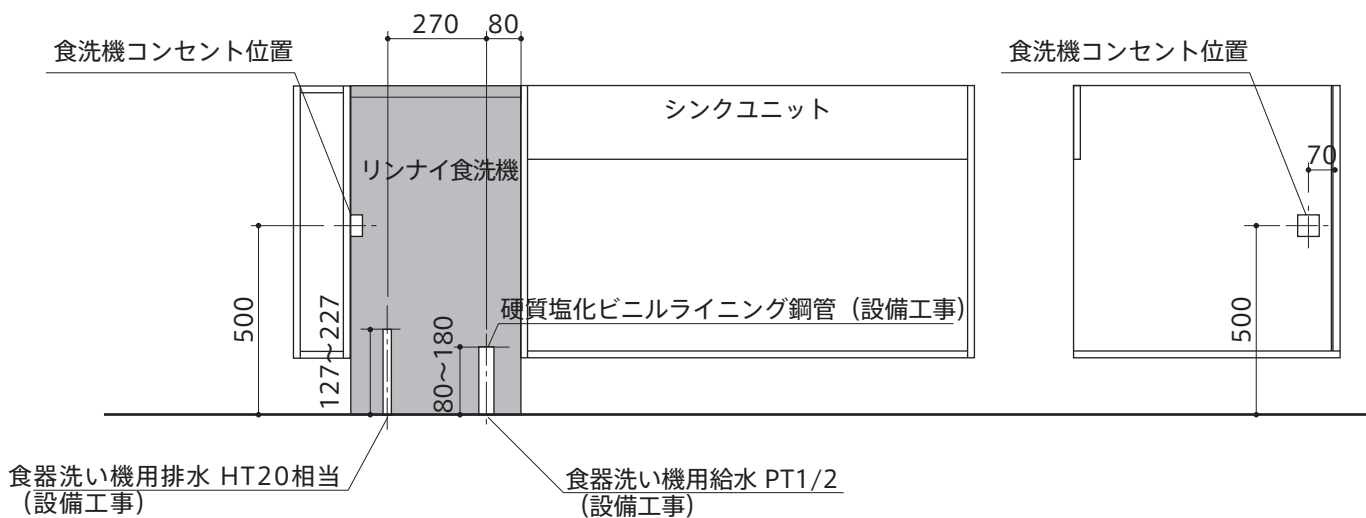
正面図
