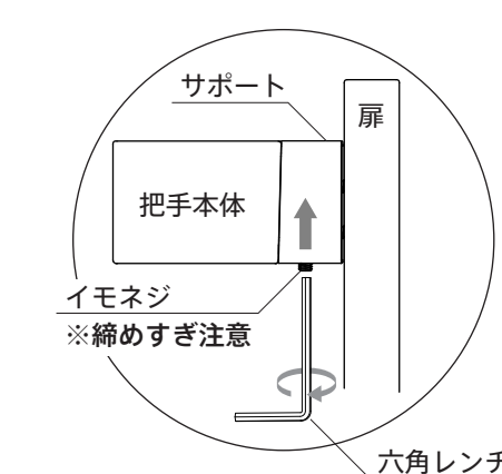
■把手本体取付断面図
