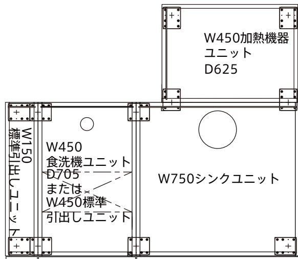
3DS/2DSシンク W1390mm×D1200mm
