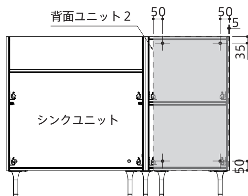
■背面ユニット2連結位置 [正面図] (前面ユニット内側からの連結位置)
