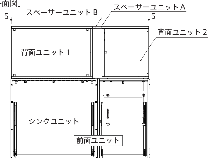
■背面ユニット2連結位置 [正面図] (前面ユニット内側からの連結位置)
