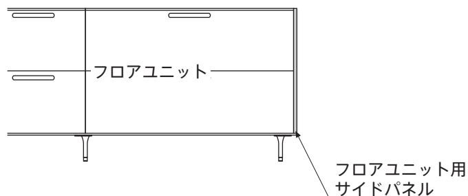
サイドパネル取付位置 (側面図)
