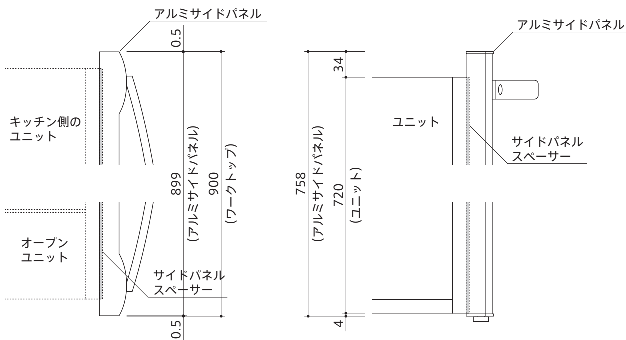
平面図
