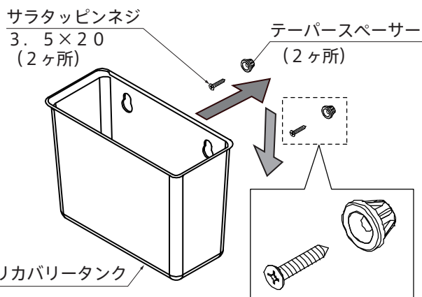
リカバリータンク取付詳細図
