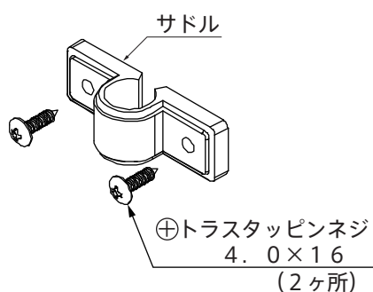
サドル取付詳細図
