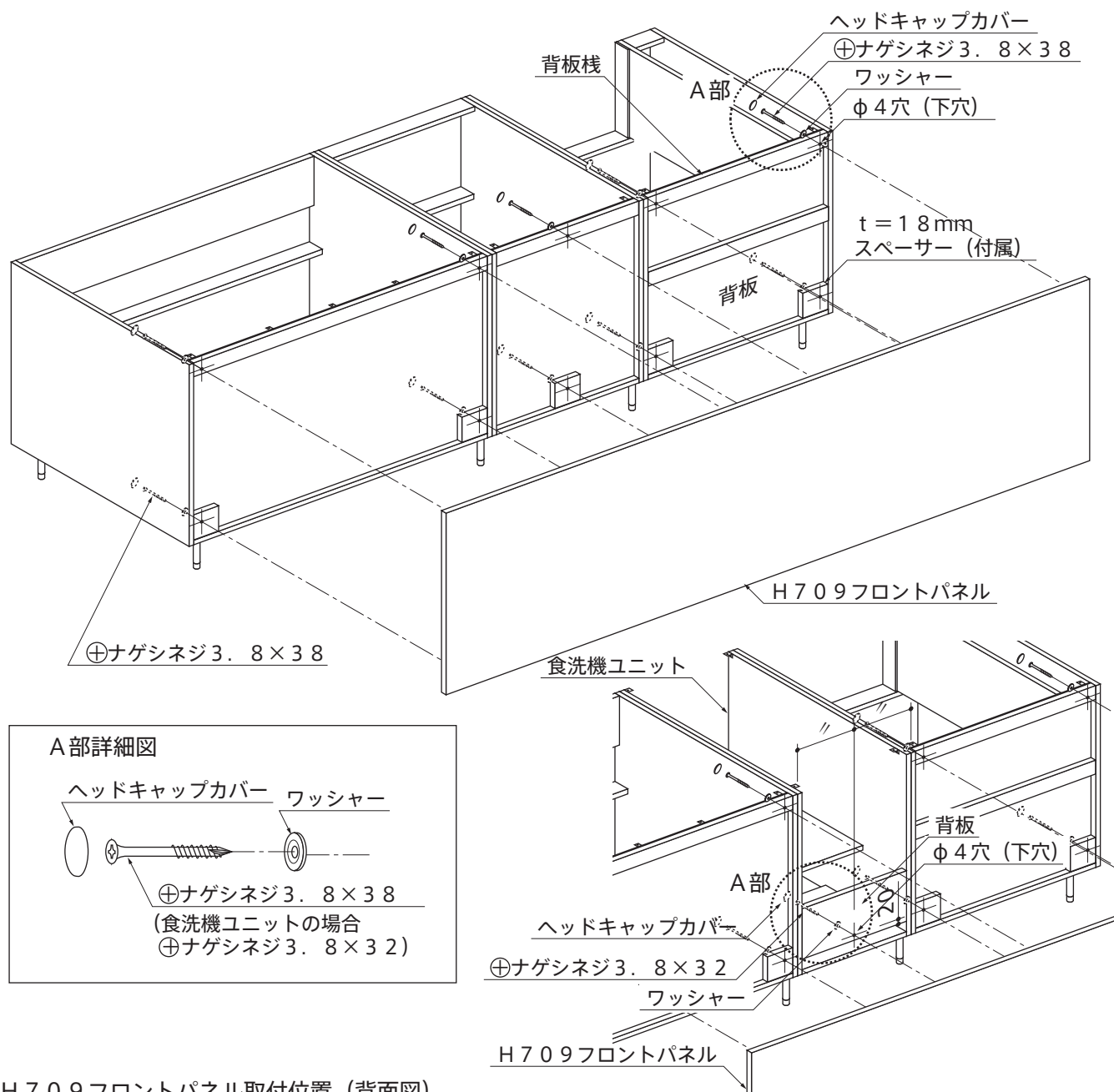
H709フロントパネル取付位置 (背面図)
