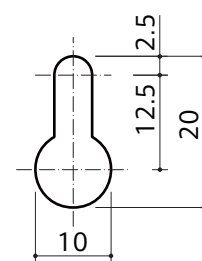
取付け穴拡大図
