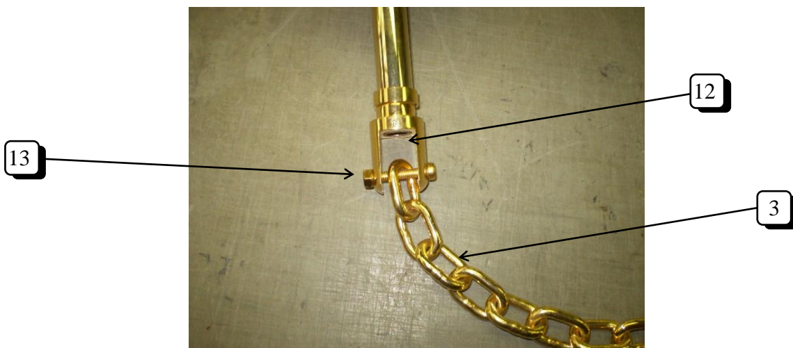
(3)チェーンを(12)シーリングベルに合わせ、(13)ネジで固定する
