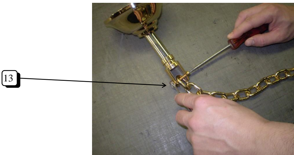
(13)ネジをしっかり締める
