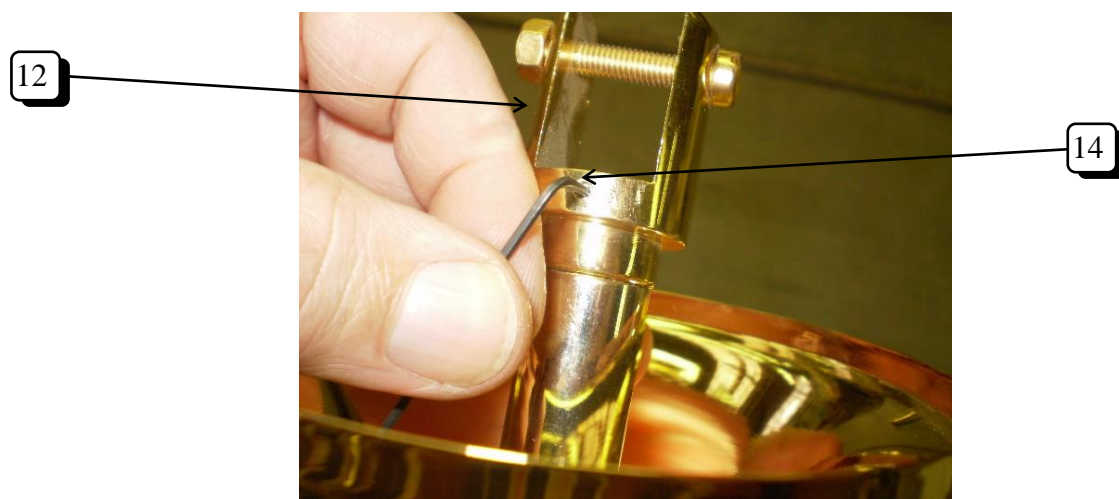
(14)シーリングベル用固定ネジで(12)シーリングベルを(11)溝付心棒にしっかり固定する
