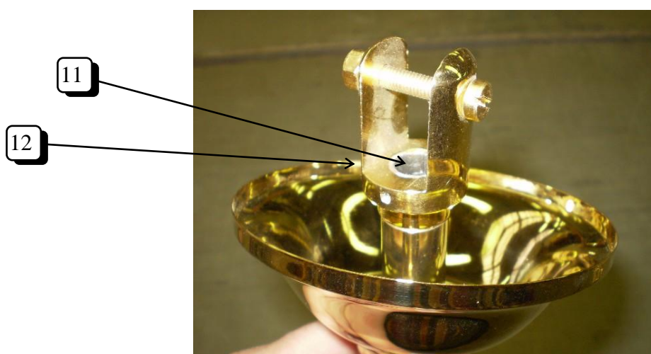
(12)シーリングベルを(11)溝付心棒に固定する
