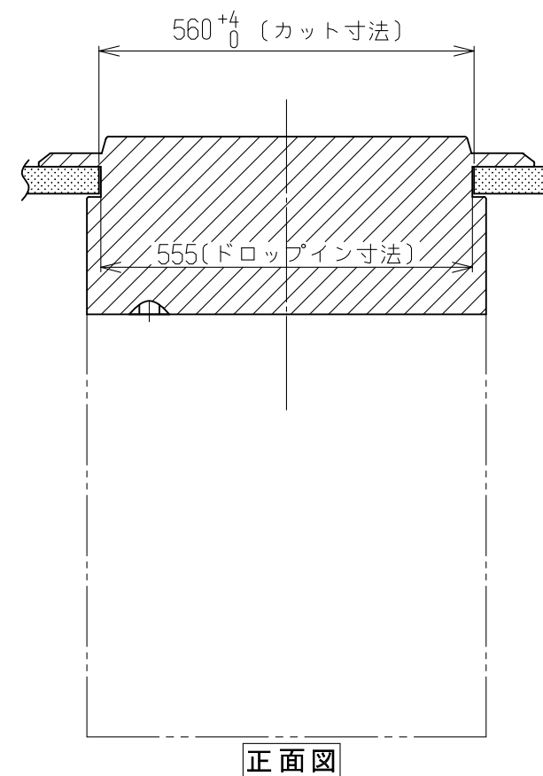
設置施工例図
