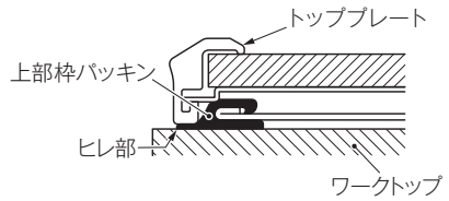
(パルクリスタルタイプ)
