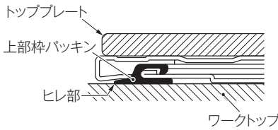
(ガラスストップタイプ)
