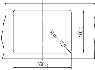
ワークトップ切り込み寸法
